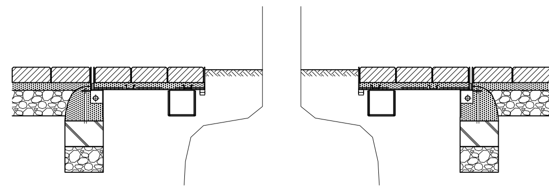
施工参考図
